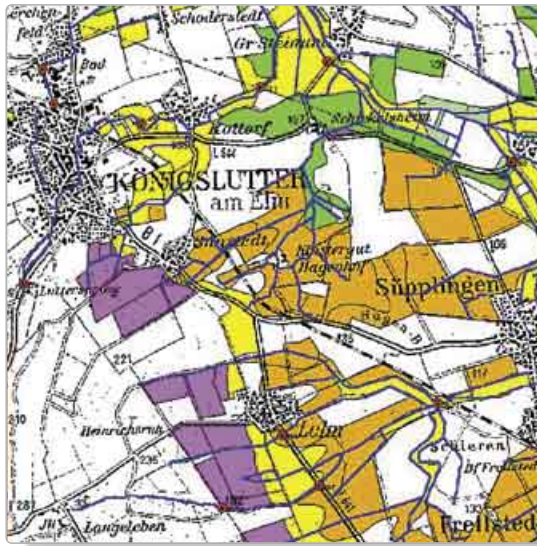
Bild 5: Berechnung der Eintragswahrscheinlichkeit von Pestiziden in Fließgewässer einer intensiv genutzten Agrarlandschaft in der Magdeburger Börde. Die Farben weisen in folgender Reihenfolge auf steigende Eintragswahrscheinlichkeiten hin: Grün, Gelb, Orange, Lila. (Quelle: Dr. Matthias Liess)
